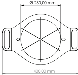
76587 Manuel Karpuz Aparatı Bıçak (6'lı) (Montajlı)
