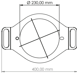
76586 Manuel Karpuz Aparatı Bıçak (4'lü) (Montajlı)
